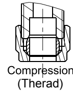
OPTIONS OF OUTLET CONNECTION OPSİYONEL ÇIKIŞ UÇLARI
