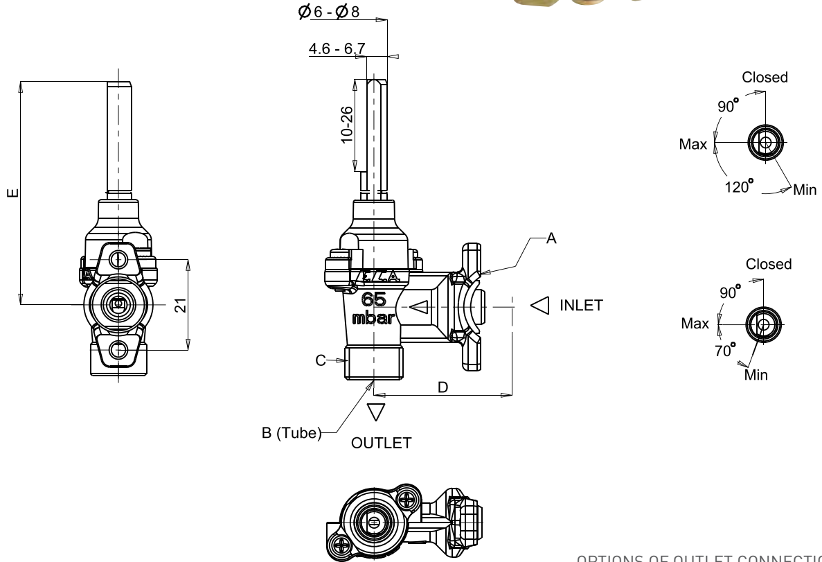
OPTIONS OF OUTLET CONNECTION OPSİYONEL ÇIKIŞ UÇLARI
