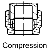
OPTIONS OF OUTLET CONNECTION OPSİYONEL ÇIKIŞ UÇLARI
