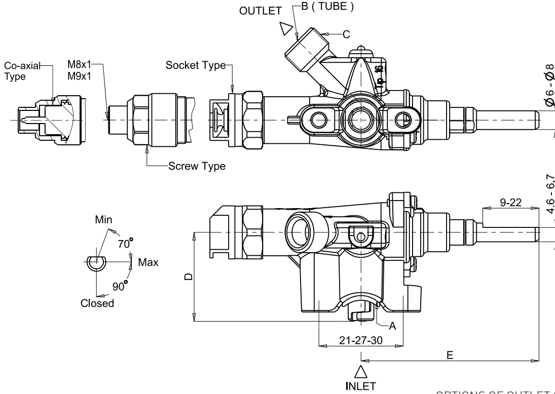
OPTIONS OF OUTLET CONNECTION OPSİYONEL ÇIKIŞ UÇLARI
