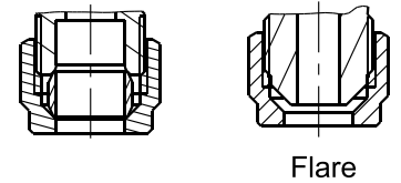
OPTIONS OF OUTLET CONNECTION OPSİYONEL ÇIKIŞ UÇLARI
