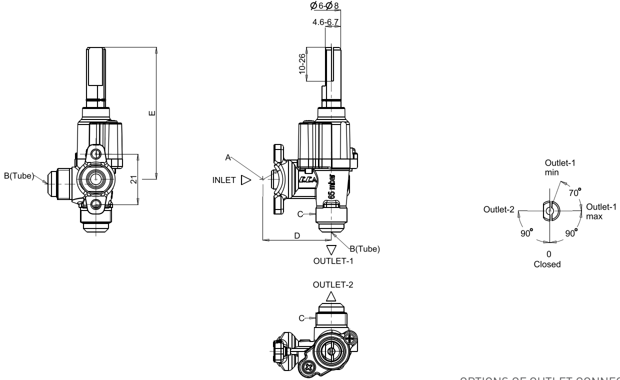
OPTIONS OF OUTLET CONNECTION OPSİYONEL ÇIKIŞ UÇLARI
